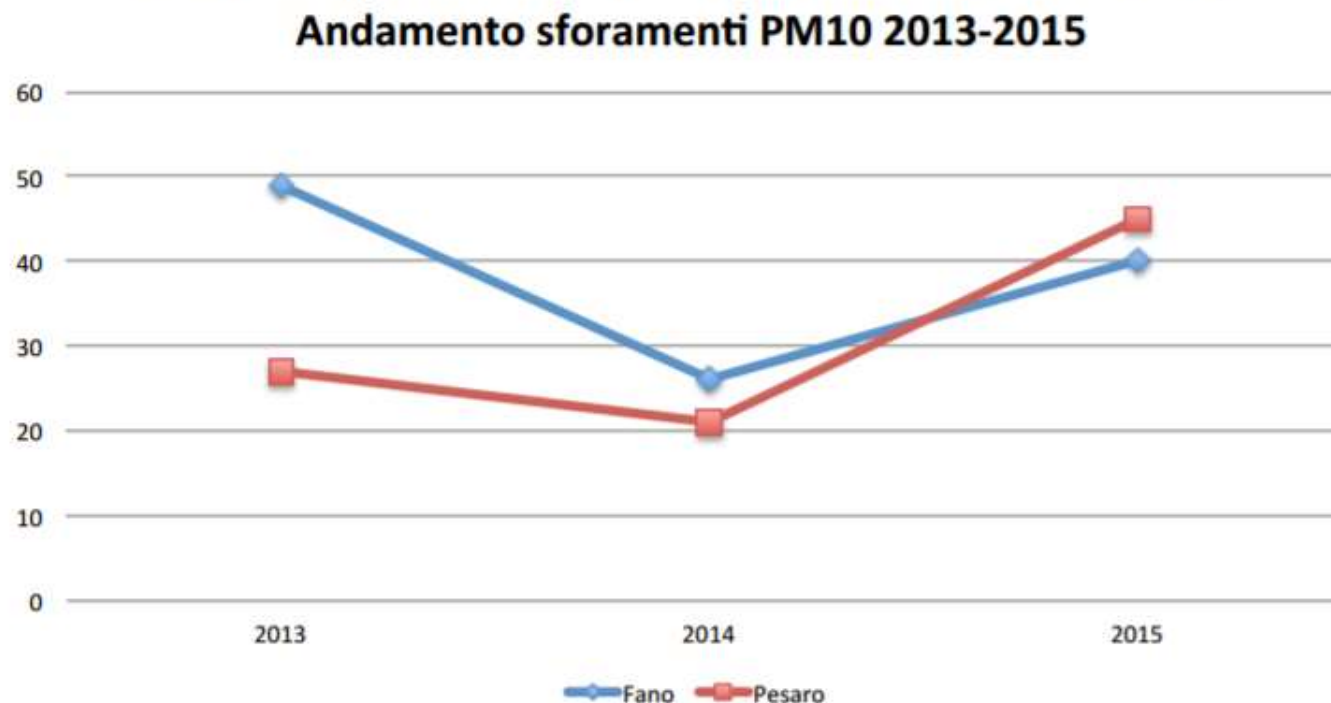
Grafico 97 – Andamento sforamenti PM10 2013-2015 (valore soglia sforamento giornaliero >50 µg/m3)
